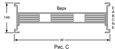
Поперечное сечение секции под отводные блоки и транспортной секции внутренней установки (IP54)
