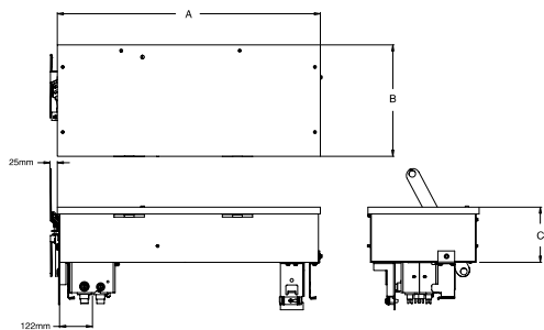
Рис. 2. Отводной блок на ток 252 - 500 А
