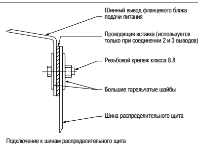
Подключение к шинам распределительного щита
